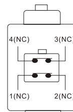
二闭型 2NC Type
